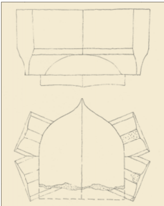
5. A szentélyboltozat nyugati zárókövének felmérési rajza
