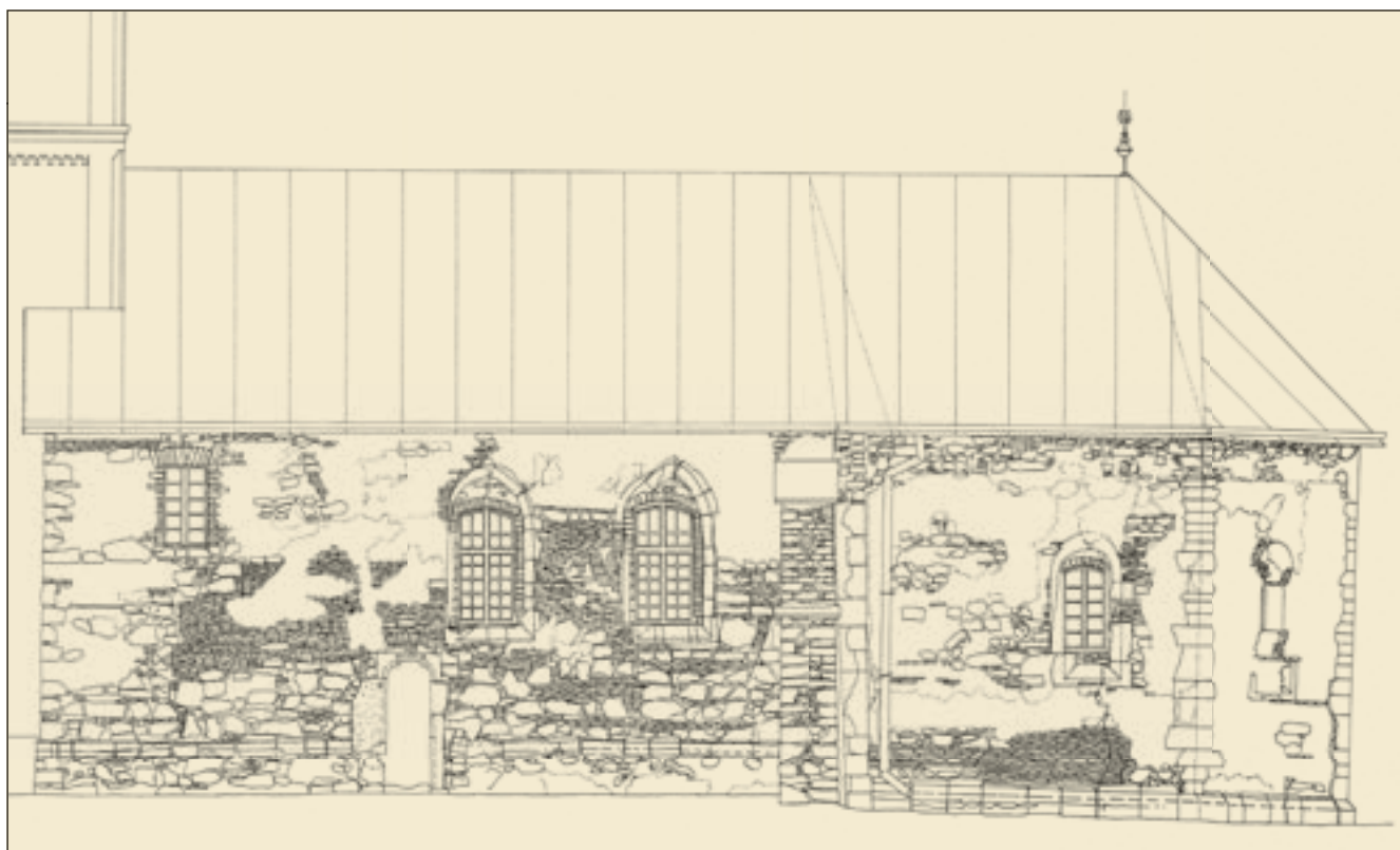
1. A déli homlokzat részlete a kutatások után
