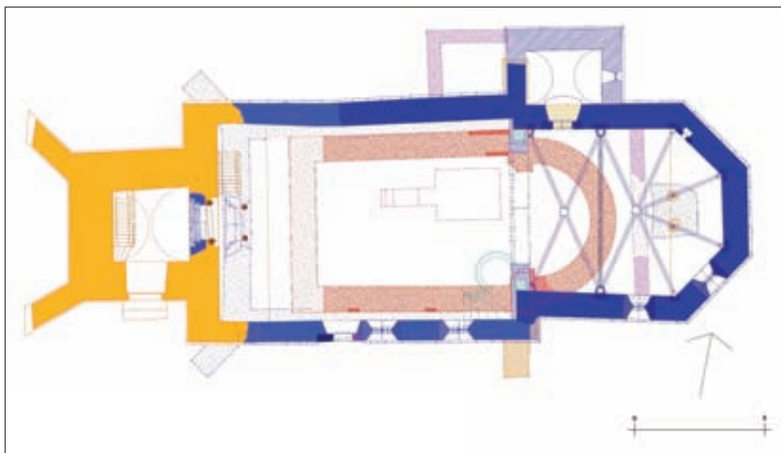
8. A templom alaprajza az építési korszakokkal
