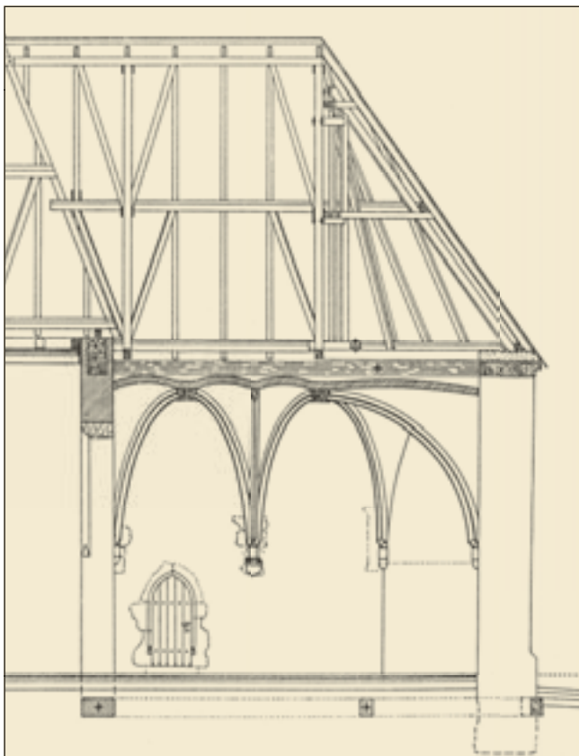
13. A szentélyboltozat rekonstrukciója, helyreállítási terv, hosszmetset, részlet
