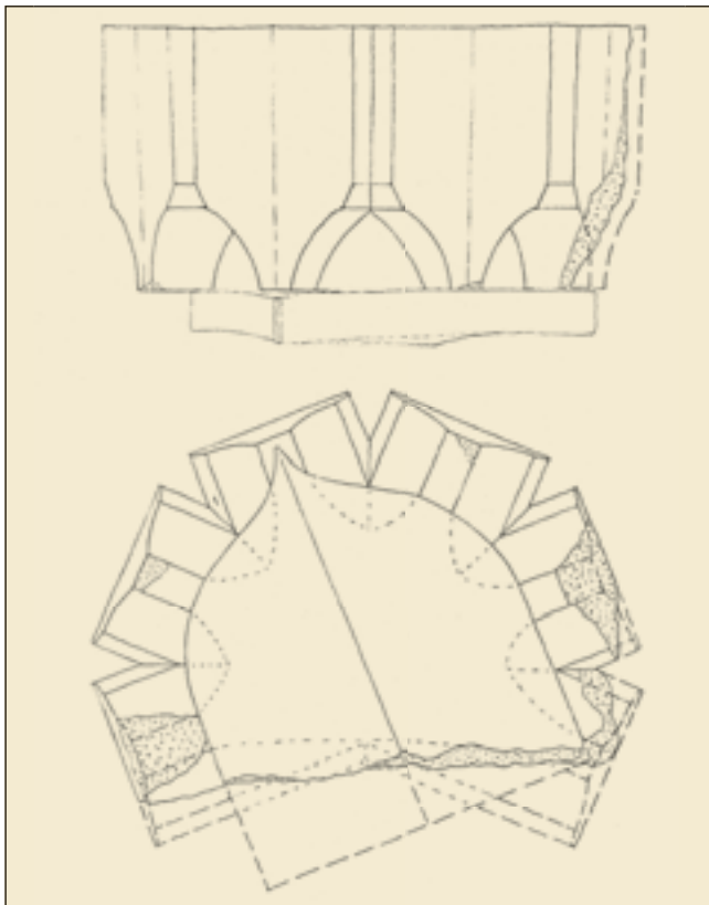
4. A szentélyboltozat keleti zárókövének felmérési rajza
