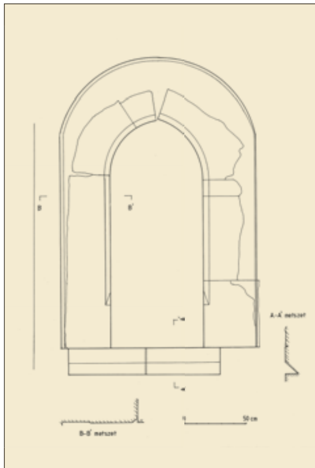
14. A sekrestyeajtó felmérési rajza
