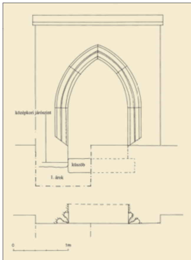
5. A déli kapu felmérési rajza
