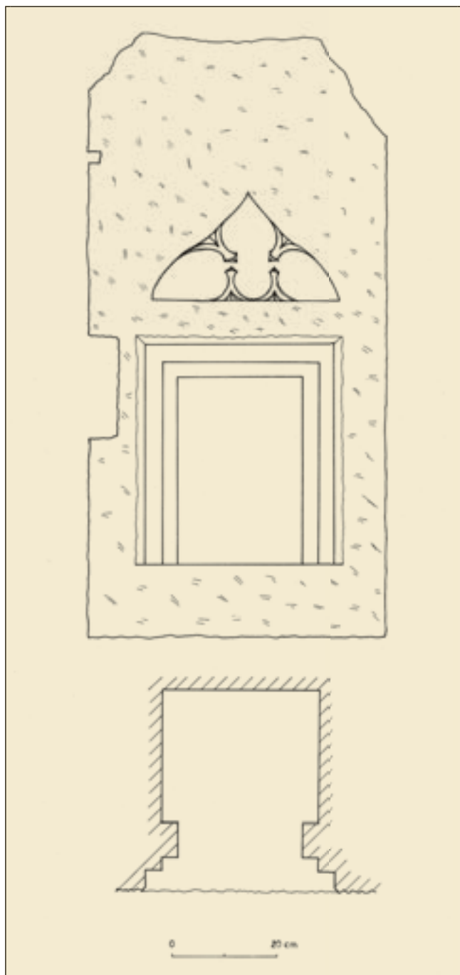
13. A szentségtartó felmérési rajza
