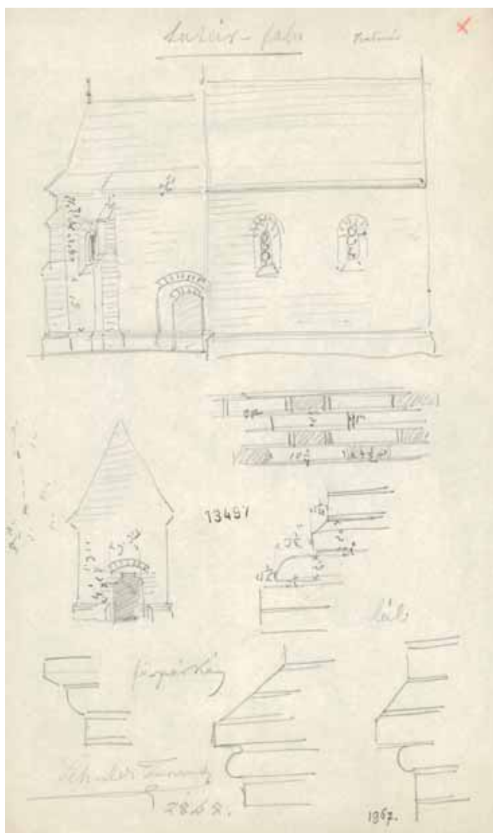
1. A templom északiként ábrázolt déli homlokzata, nyugati nézete és párkányrészelei, Schulcz Ferenc, 1864
