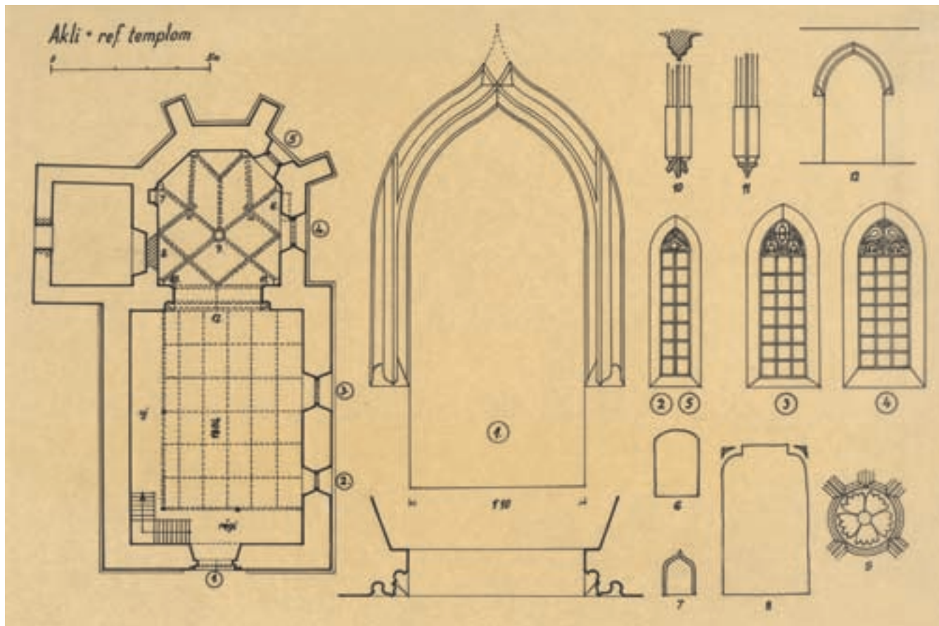
3. A templom alaprajza részletrajzokkal (Várnai Dezső, 1940)
